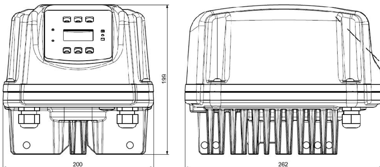
Afbeelding1: aanzicht en afmetingen
