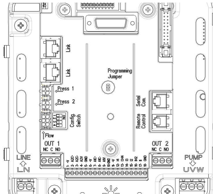
Afbeelding 5: aansluitingen
