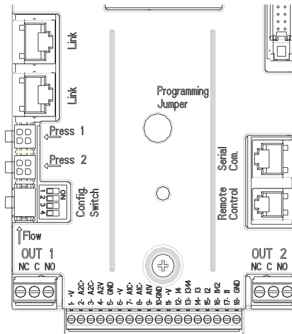
Afbeelding 5: aansluitingen
