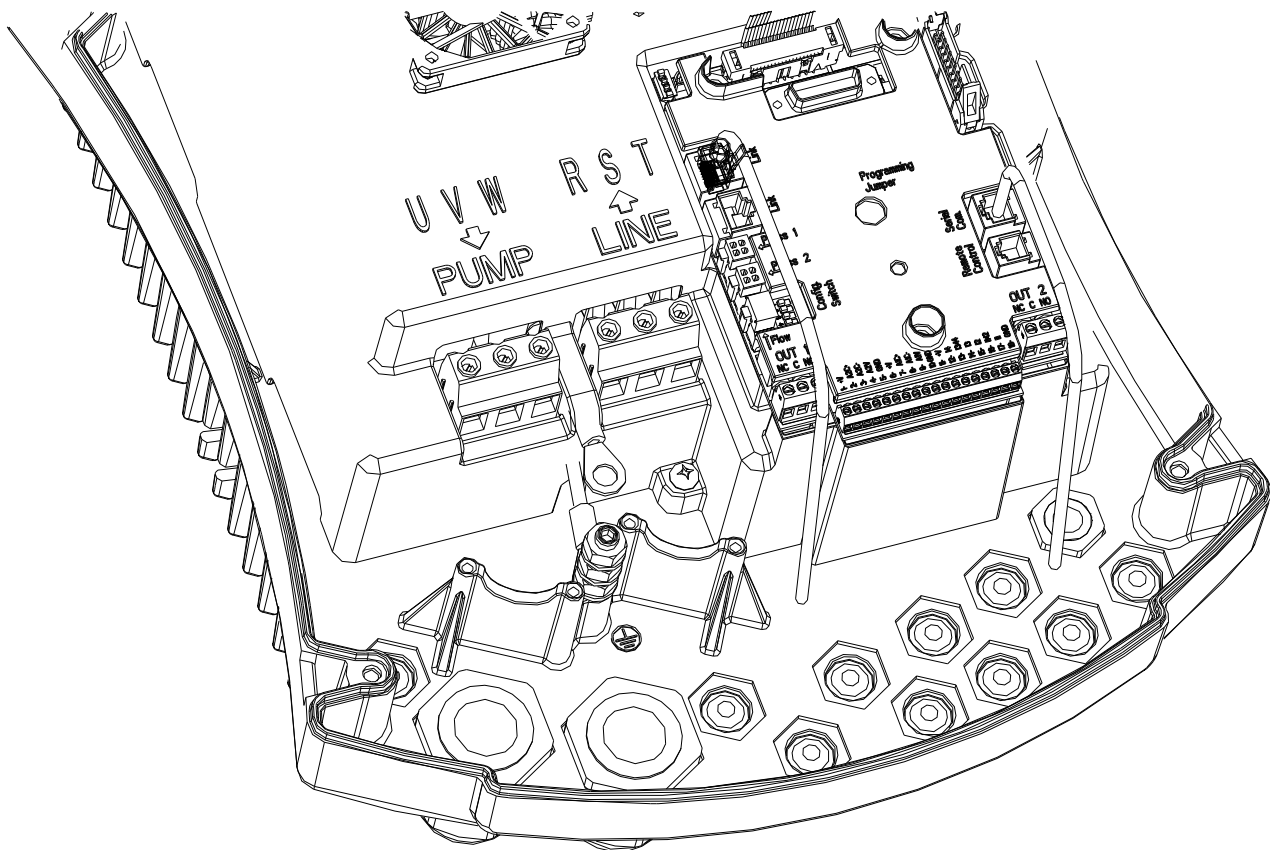
Afbeelding 2: Elektrische aansluitingen
