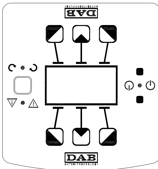
Afbeelding 7: Bedieningspaneel
