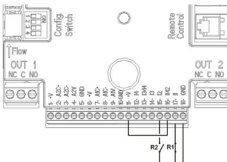
Afbeelding 4: Aansluitvoorbeeld digitale ingangen
