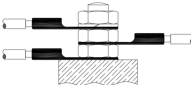
Afbeelding 2: Aardaansluiting
