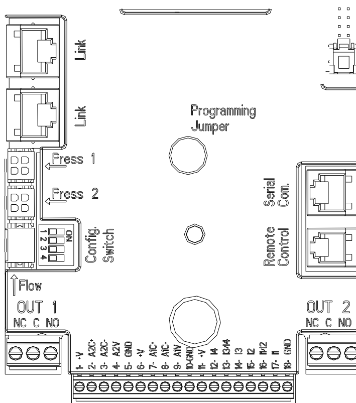
Afbeelding 3: Aansluitingen
