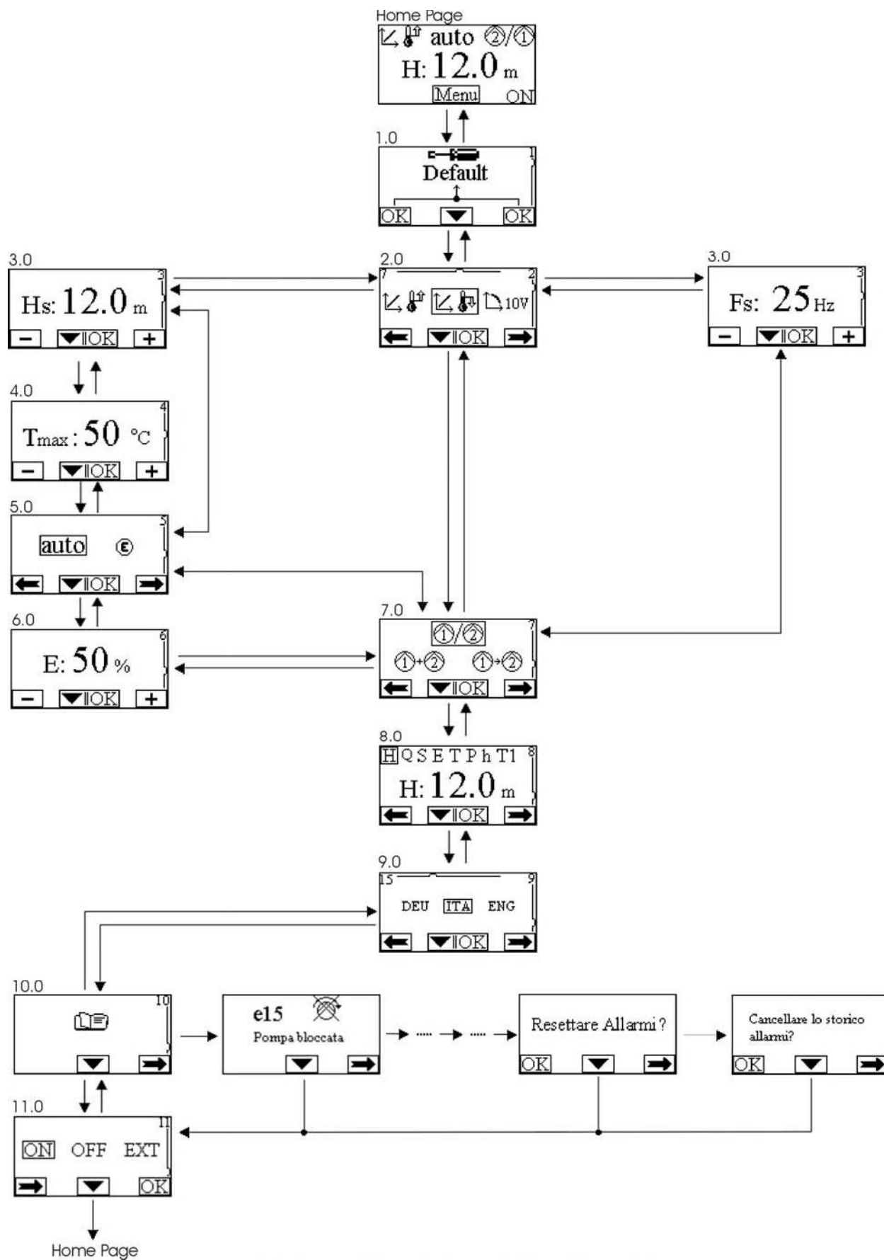
Afbeelding 8: Menu MCE/C
