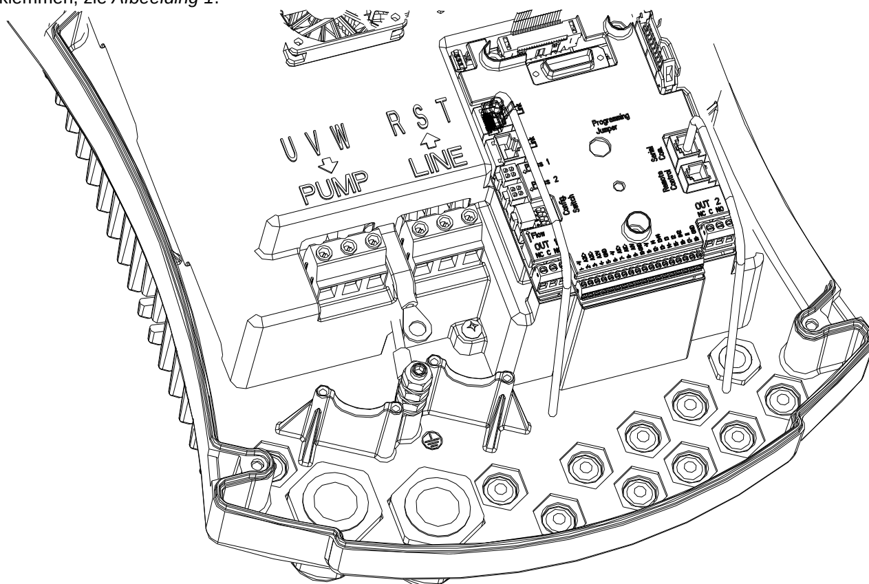
Afbeelding 1: Elektrische aansluitingen
